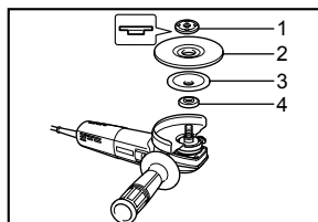
1. Contratuercas 2. Disco flexible 3. Plato de goma 4. Brida interior
