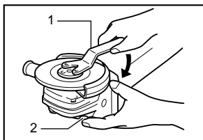
1. Llave de tuercas 2. Bloqueo del eje
