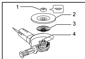
1. Contratuercas 2. Disco para esmerilar de centro hundido / multidisco 3. Brida interior 4. Eje
