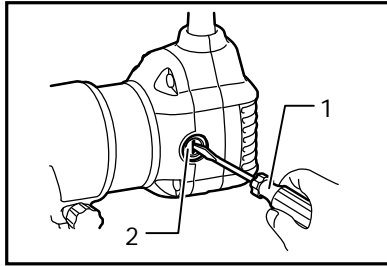
1. Destornillador 2. Tapa del carbón
