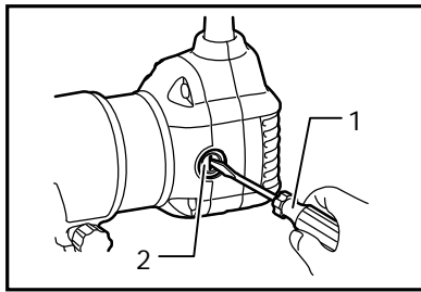
1. Tournevis 2. Bouchon de porte-charbon
