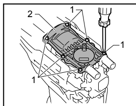
1. Tornillos 2. Tapa del cárter
