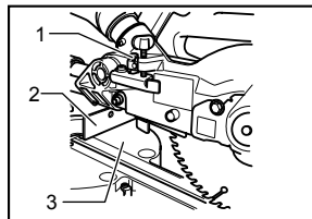
1. Boulon de réglage 2. Garde de guidage 3. Socle rotatif
